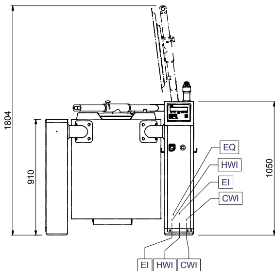
Zij aanzicht
